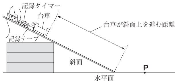
図3 実験装置
