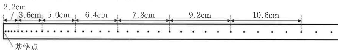
図 5 斜面の傾きが 20^\circ のときの記録テープ
