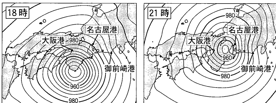
図1 ある日の18時と21時の地上天気図
