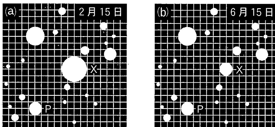
図2 図1の右図の領域における天体像の時間変化
