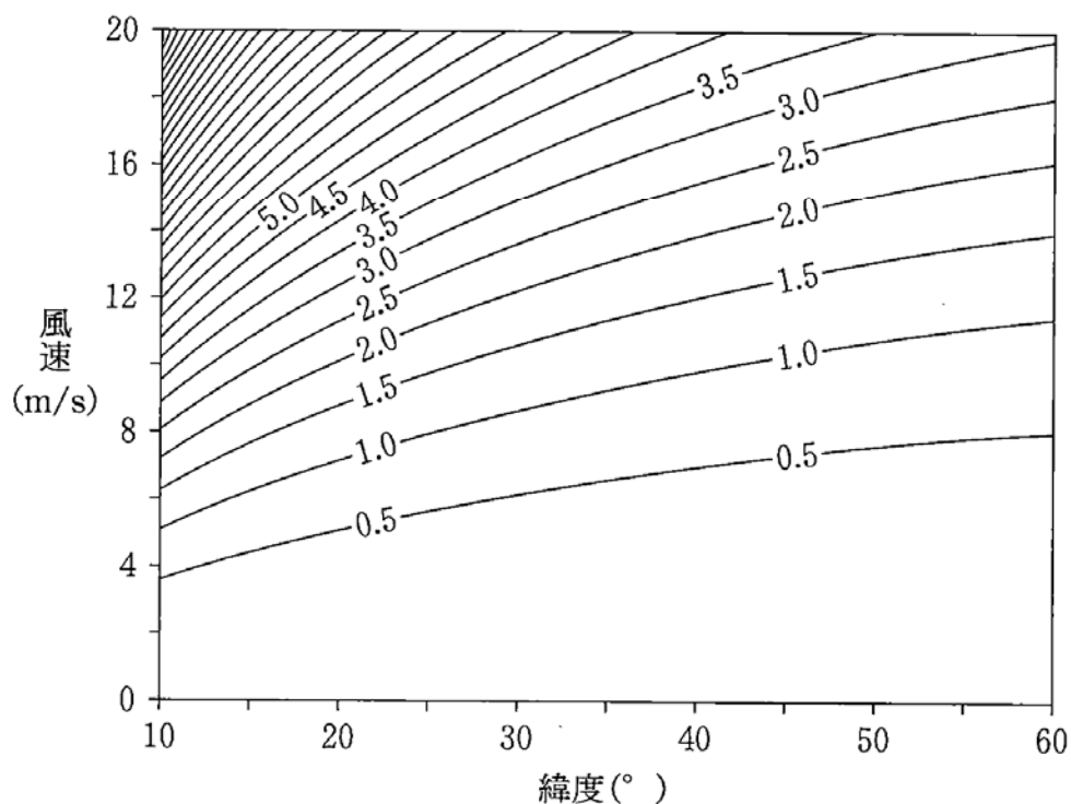
図3 エクマン輸送量 ( \text{m}^2/\text{s} ) の風速と緯度に対する依存性 等値線はエクマン輸送量を示す。
