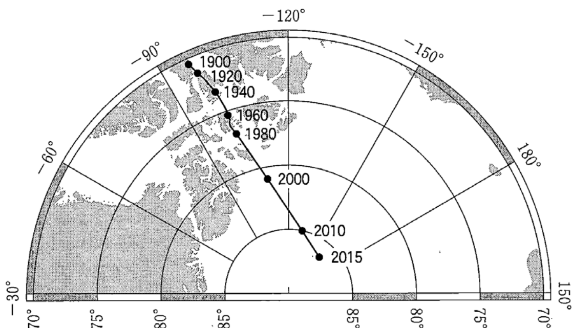
図 1 1900～2015 年の磁北極の移動曲線
