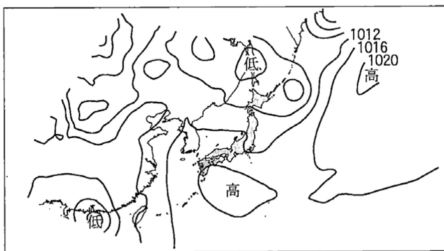
図1 地上天気図
