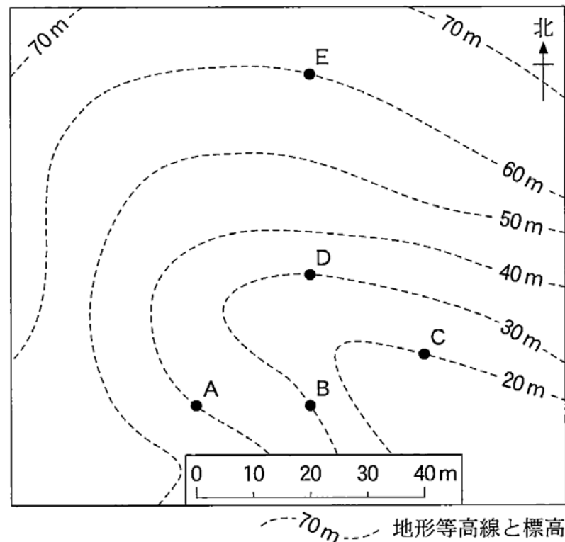
図2 ある地域の地形と露頭の位置
