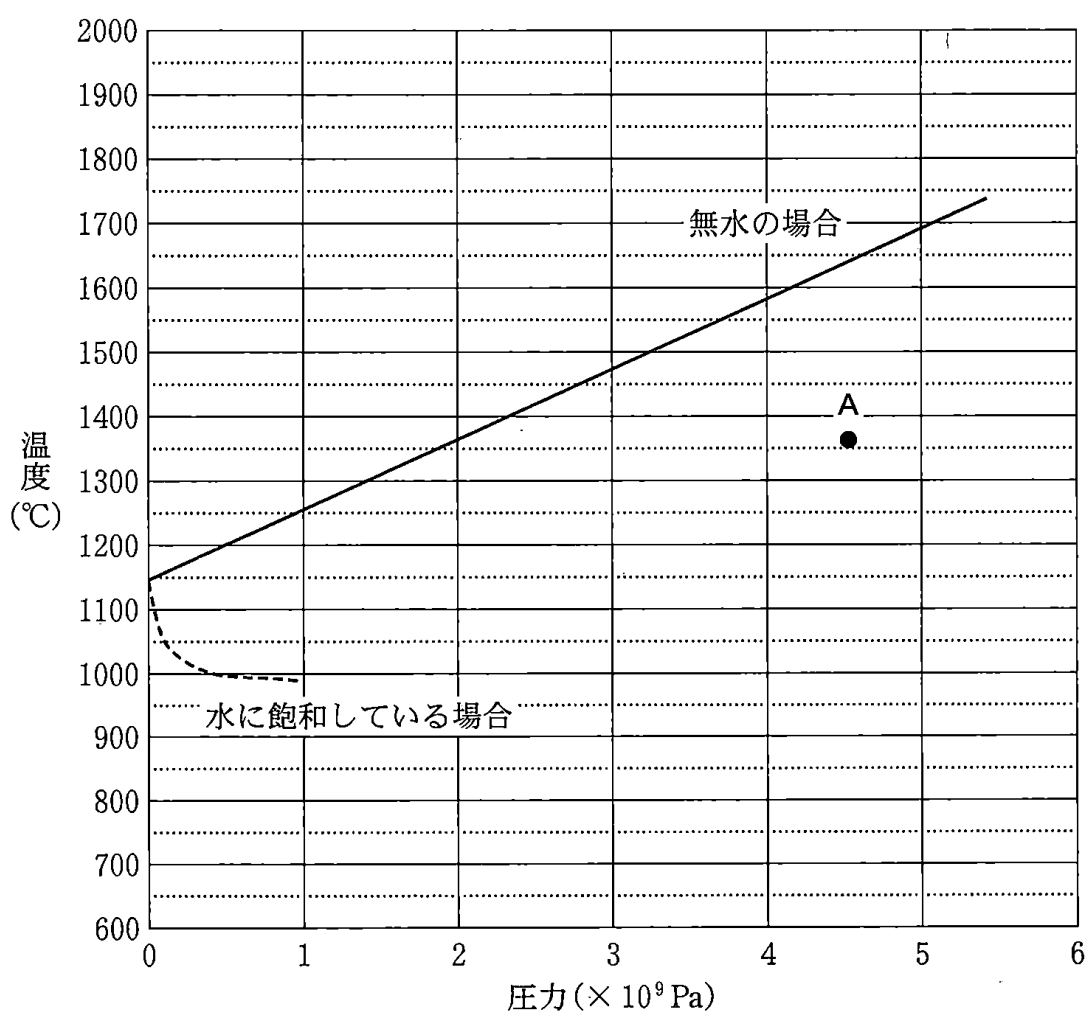
図 3 マンツル物質の融解曲線
