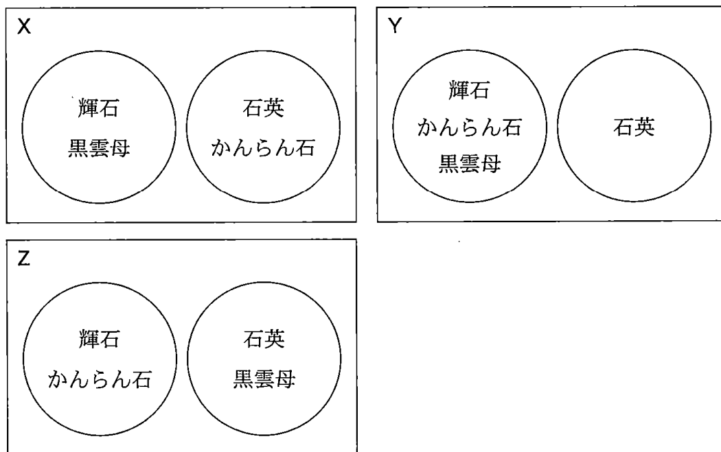
図1 鉱物のグループ分けの図
