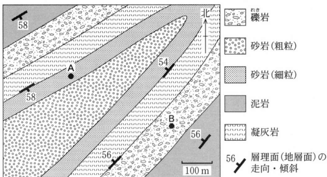
図5 ある平坦な地域の地質図
