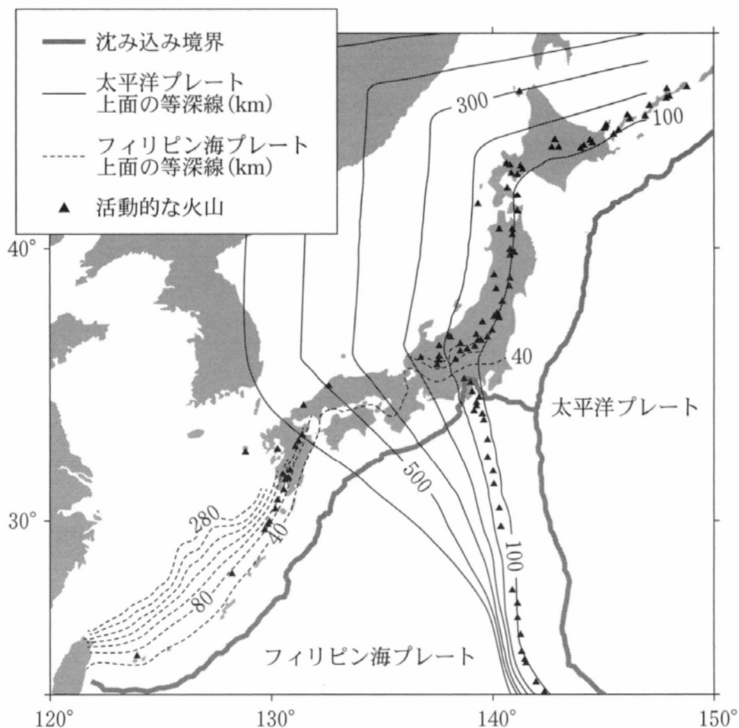
図 2 日本周辺のプレートと活動的な火山の分布
