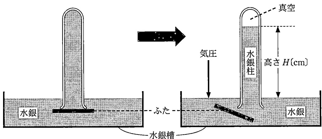
図1 気圧の測定実験の概念図
