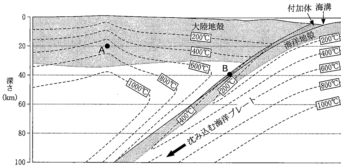
図4 沈み込み帯の温度構造を示した模式断面図(1000℃ 以上は省略)
