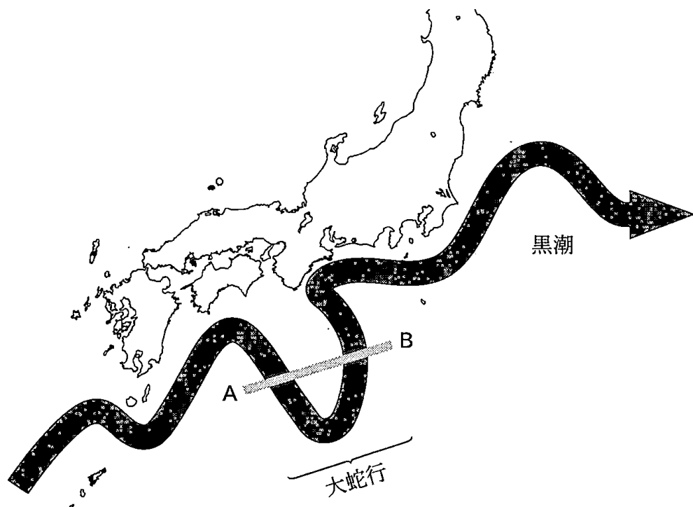
図3 2017年8月に発生した黒潮の大蛇行
