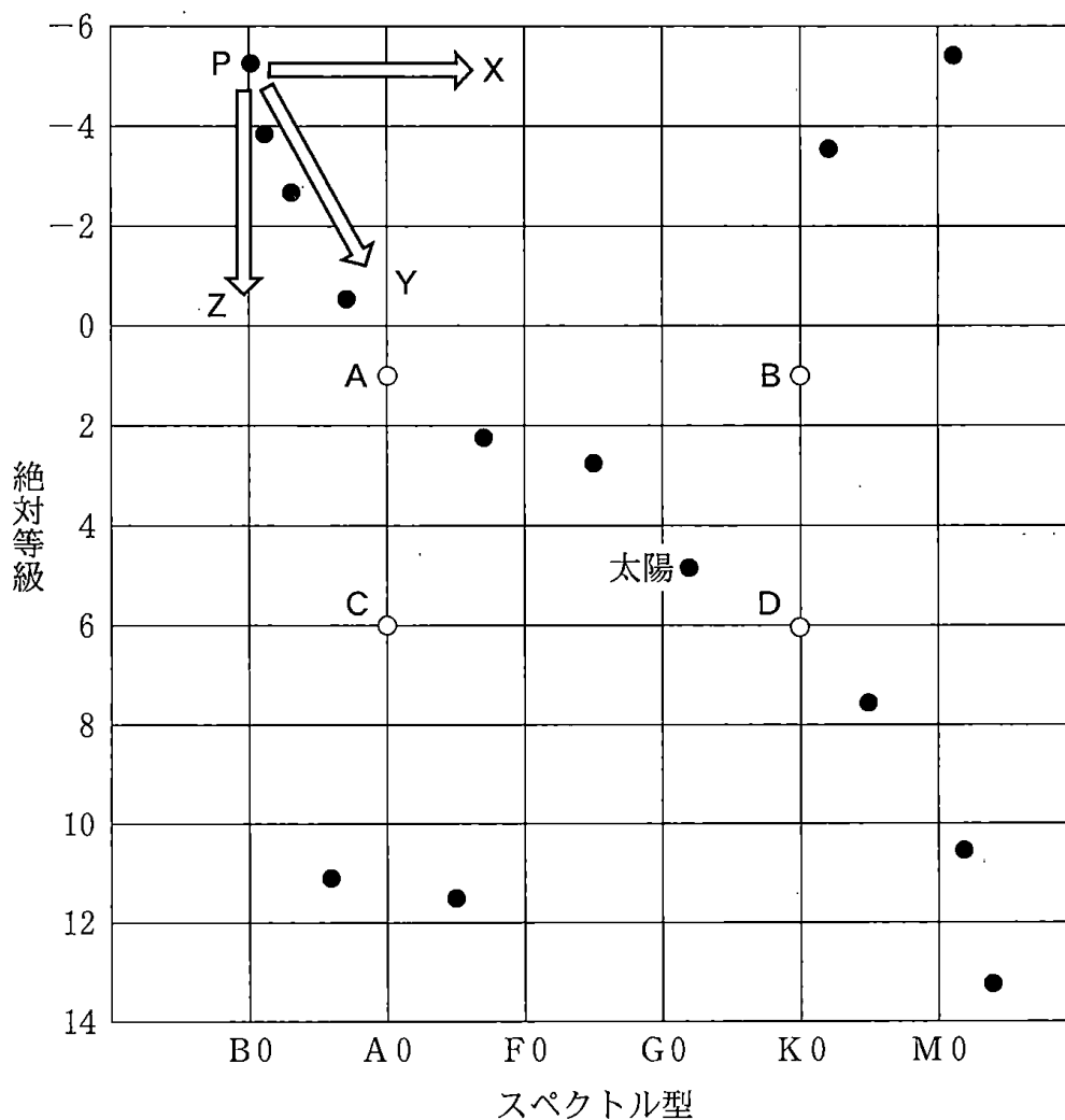
図2 Sさんが作成したHR図
