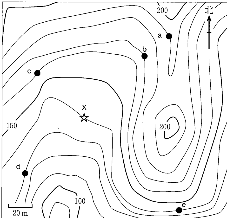
図 5 ある地域の地形図と調査地点の位置
