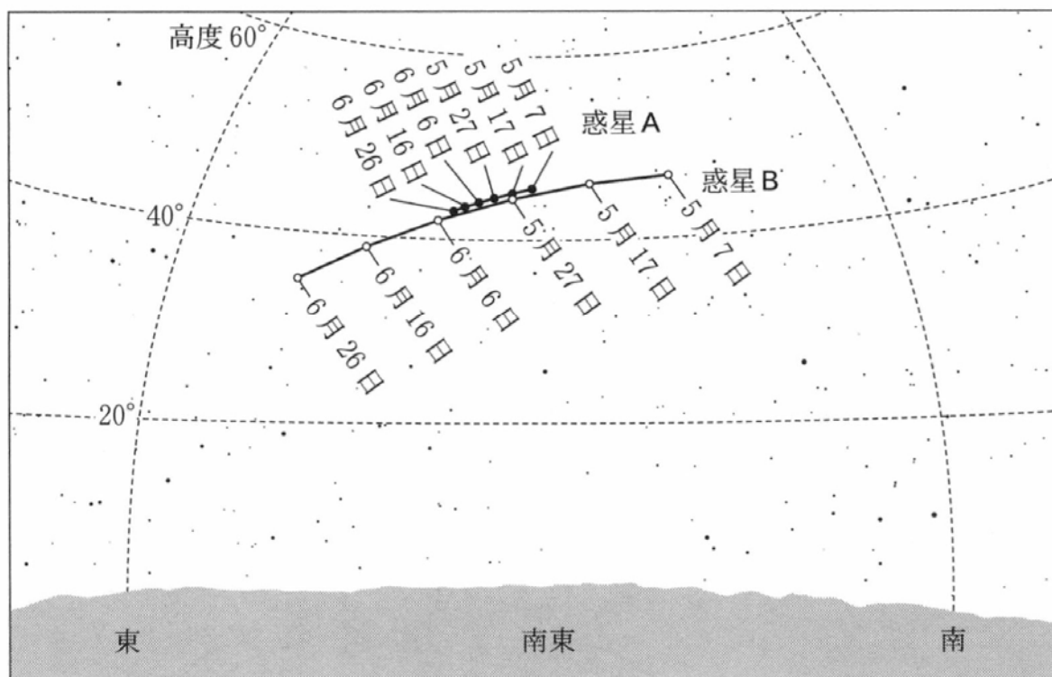
図1 惑星の動き
