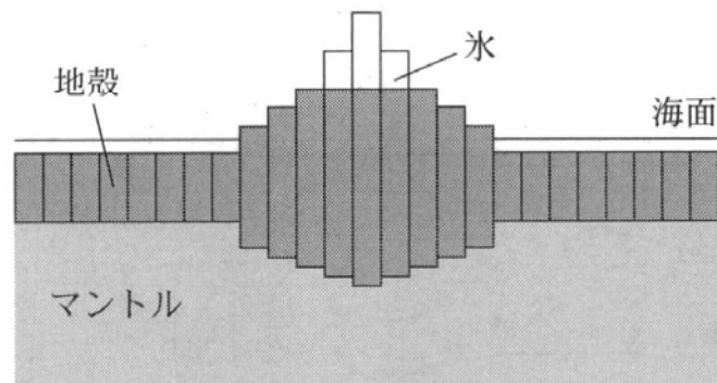
図1 氷がとける前の地下構造
