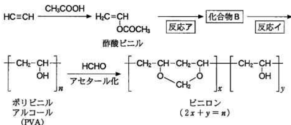
図1 ビロンの合成経路
