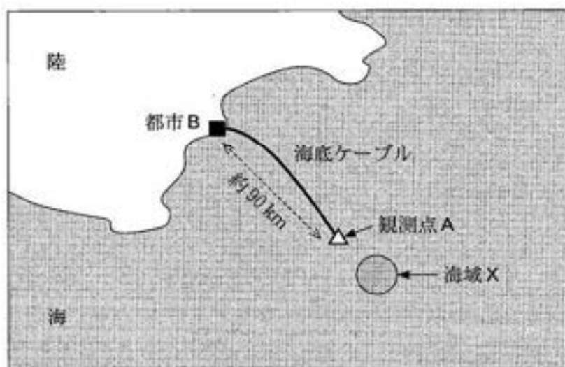
図 1 津波観測システムの概略図
