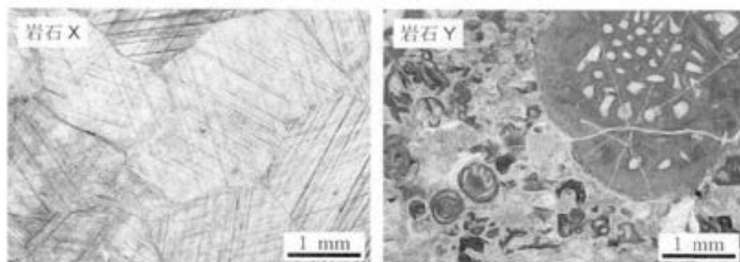
図 3 偏光顕微鏡写真(開放ニコル)
