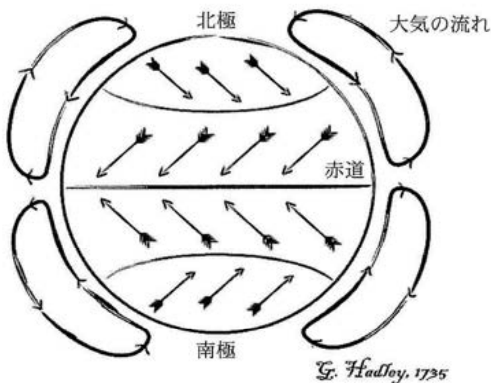
図 2 ハドレーが考えた大気の大循環の概念図 矢印は大気の流れを示す。
