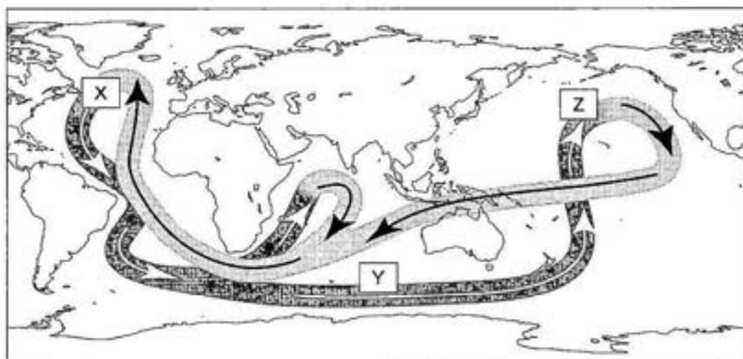
図 4 コンベアベルトの概念図と海域 X～Z
